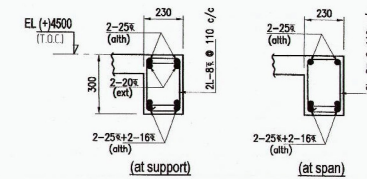
DET. OF SB-1(230x300)
